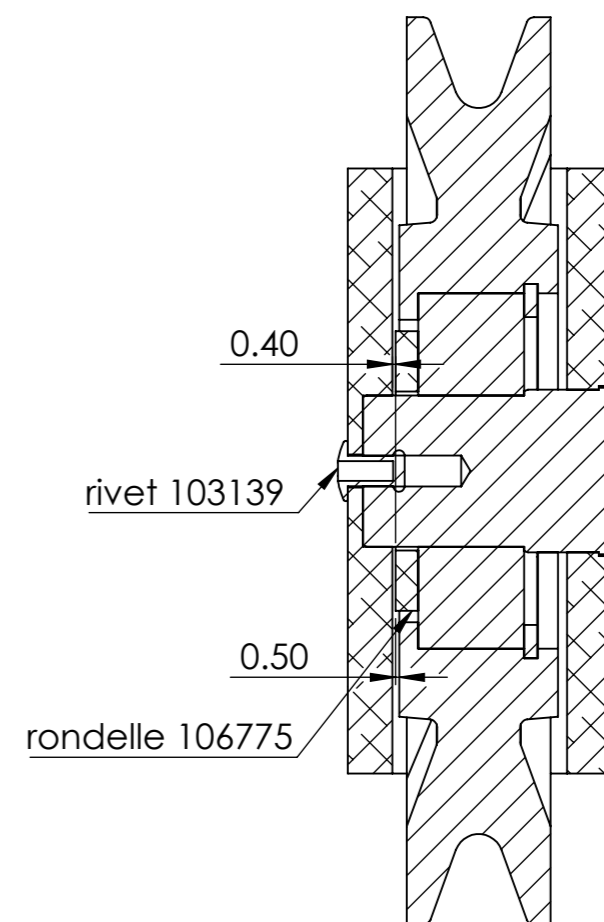
COUPE A-A
