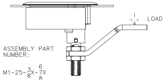
LONG PAWL
