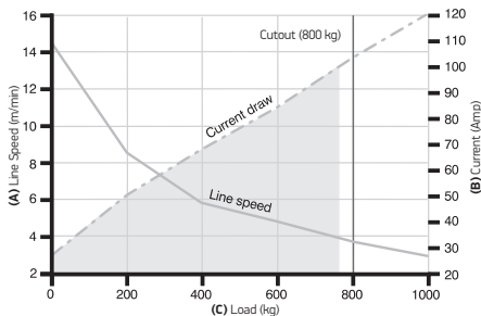
OCEAN 46 + EVO™ 45 - 24V
